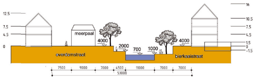
doorsnede A-A'
